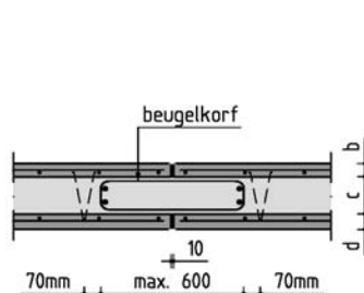
Detail H2 - principedetail plaatvoeg
