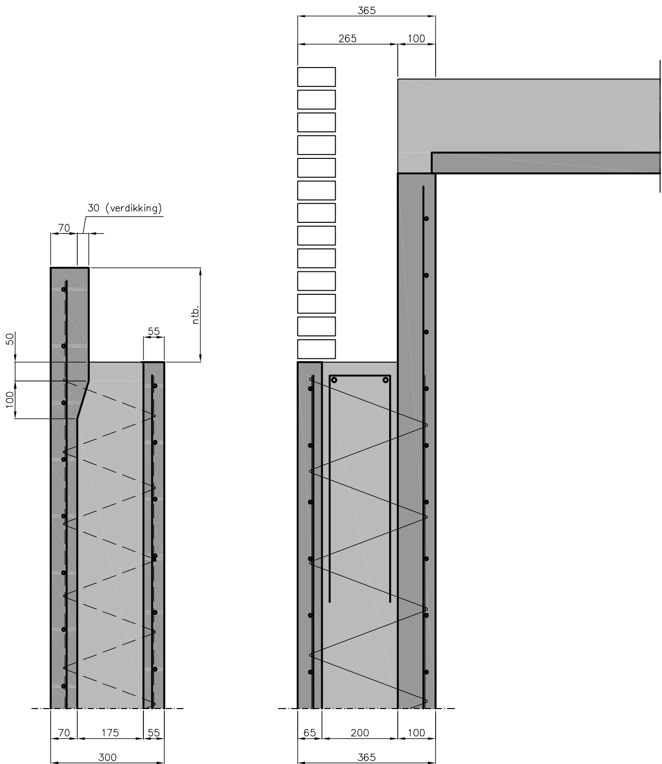
Principedetails dragende schillen Schaal 1:10
